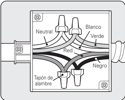
Caja de conexiones
